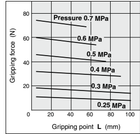
MHZ2-32S
